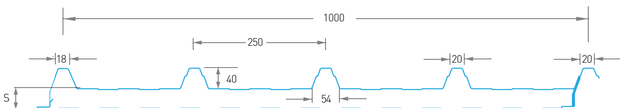
DISEGNO TECNICO PENTA
